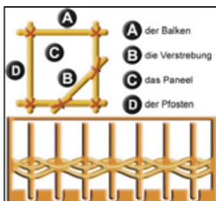
Gefach eines Fachwerkhause Zeichnung G. Tosca (LMZ RP)
