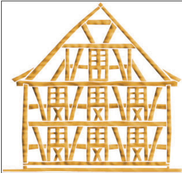
Fassade und Giebel eines Fachwerkhause Zeichnung G. Tosca (LMZ RP)
