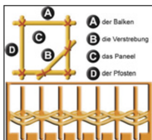
Fabrication d'un panneau Dessin G.Tosca (LMZ RP)
